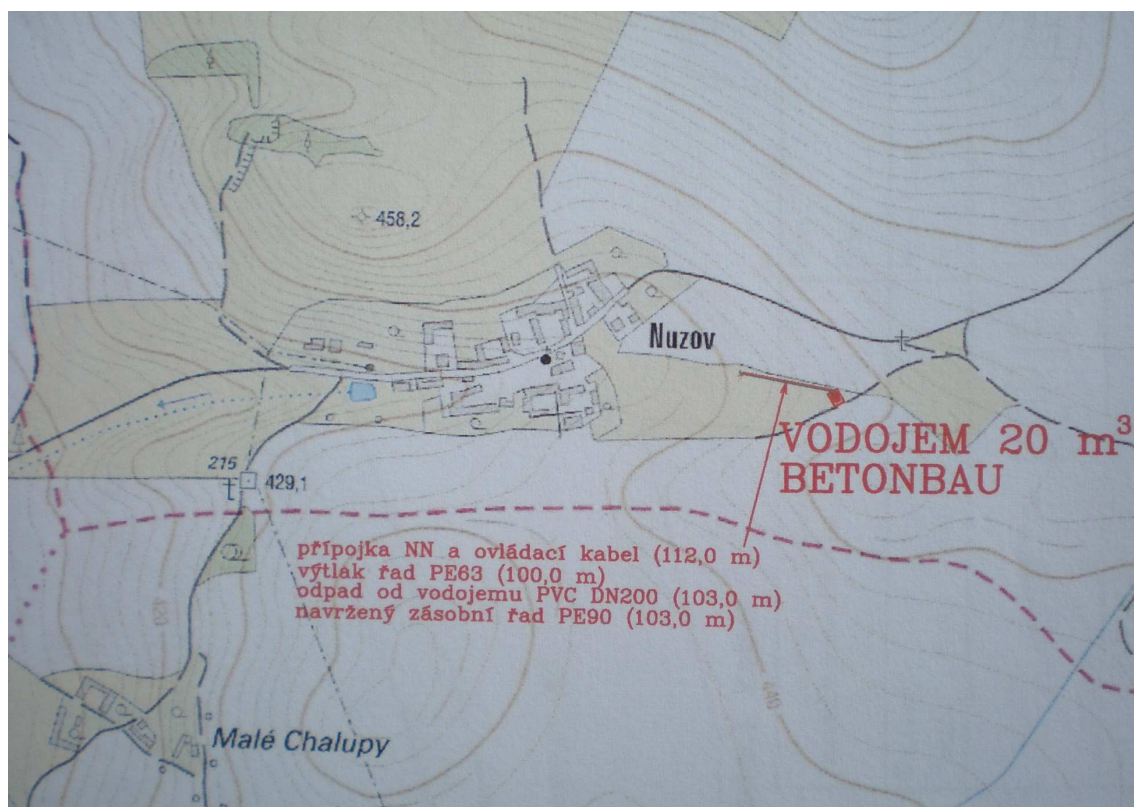
Plánovaný vodovod s vodojemem v obci Nuzov
