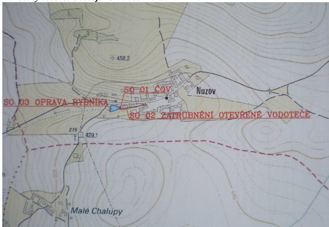
Plánované vedení a umístění ČOV v Nuzově
